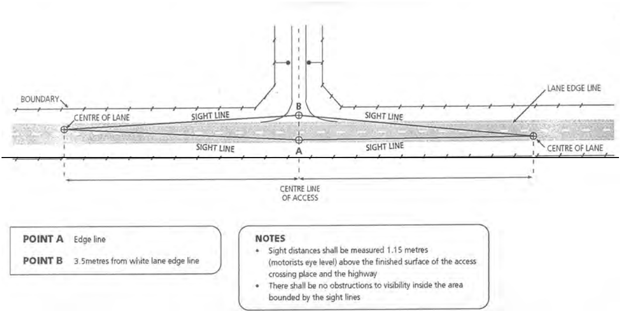
Diagram E10.A1 – Sight Distances
